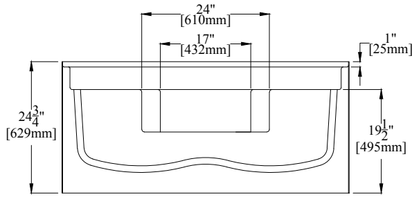
ELEVATION
